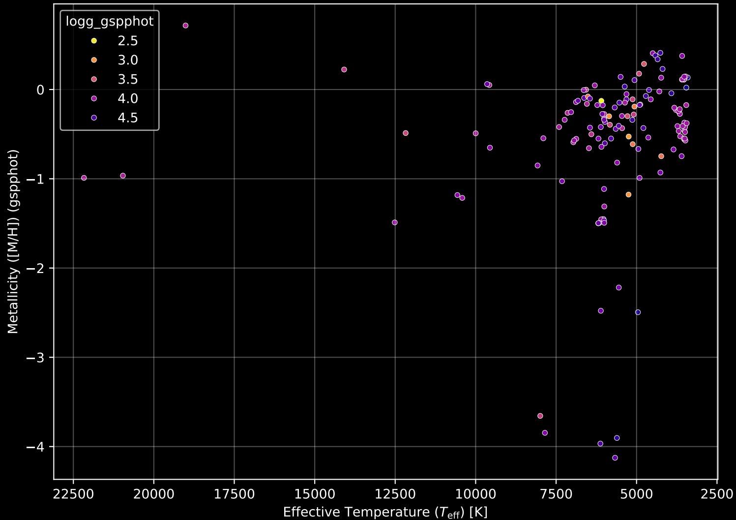
APOGEE DR17 Field: [ORIOND] Stellar Population Parameters (n= 141)
